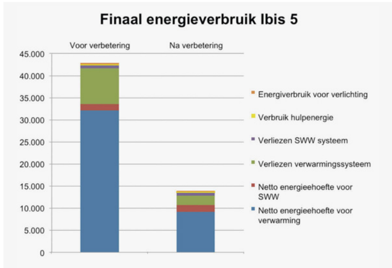
Afb. 7 Besparingen Ibissenstraat 5. Primair energieverbruik (© Cenergie).
