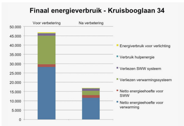
Afb. 8 Besparingen Kruisbooglaan 34. Primair energieverbruik (© Cenergie).
