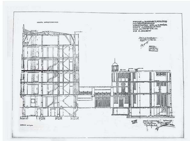
Fig. 10a et 10b Maison de rapport et fabrique de cigarette de Camille Gosset, rue Lambert Crickx à Anderlecht [arch. J. Ghobert]. Plan et coupe. Demande d'autorisation de bâtir, 1912, Anderlecht - Travaux publics.
